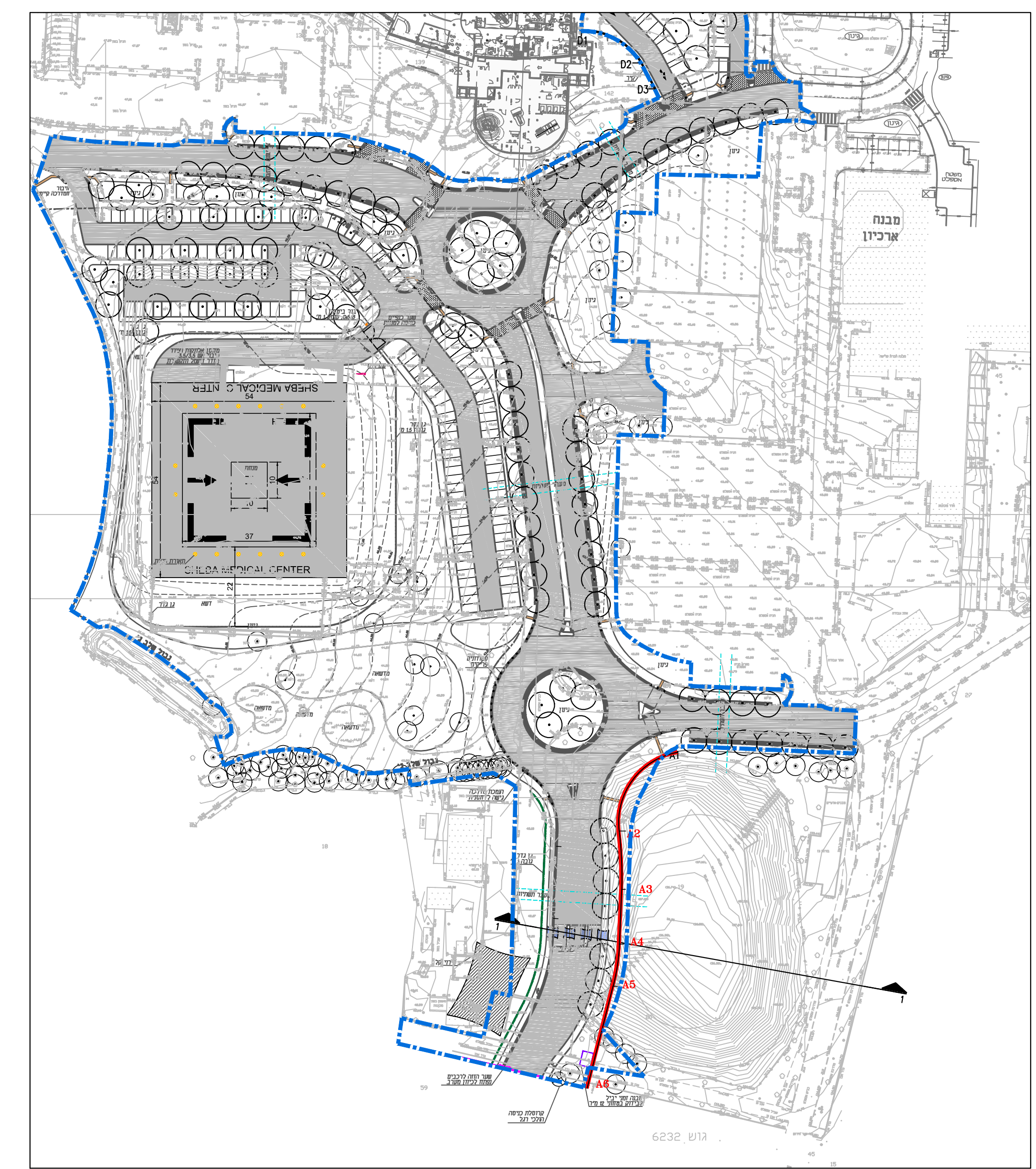
תכנית קני"מ 1:1000
